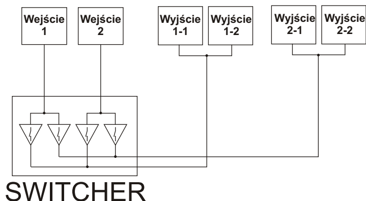
Schemat blokowy
